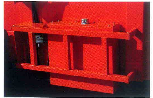
Option : Groupe hydr. entraînement tablier - diviseur électronique de débit
